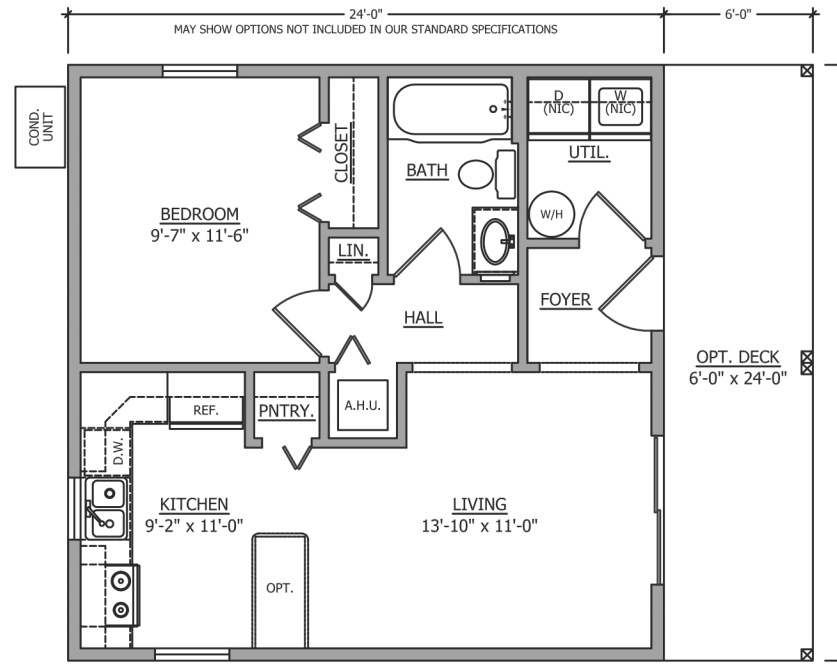
FLOOR PLAN N.T.S.
